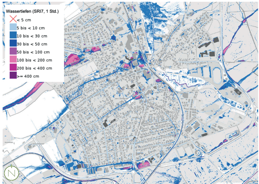
Auszug Sturzflutgefahrenkarte Ramstein; Quelle: Sturzflutgefahrenkarte Rheinland-Pfalz; https://wasserportal.rlp-umwelt.de/servlet/is/10360/
