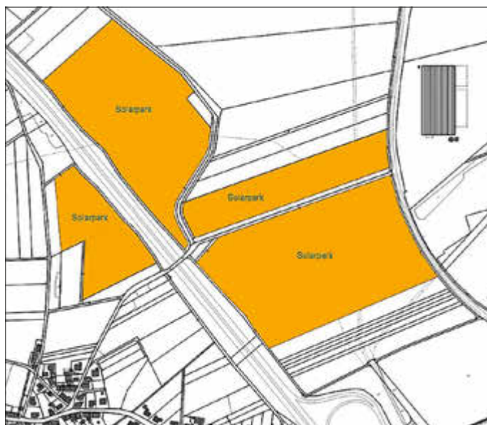
Geplante Freiflächen-PV-Anlagen entlang der A62, Gemarkung Katzenbach (Darstellung der Bauverwaltung der VGV).
